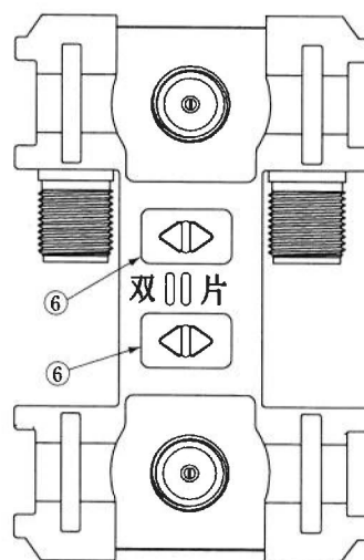
パネル未装着状態図
