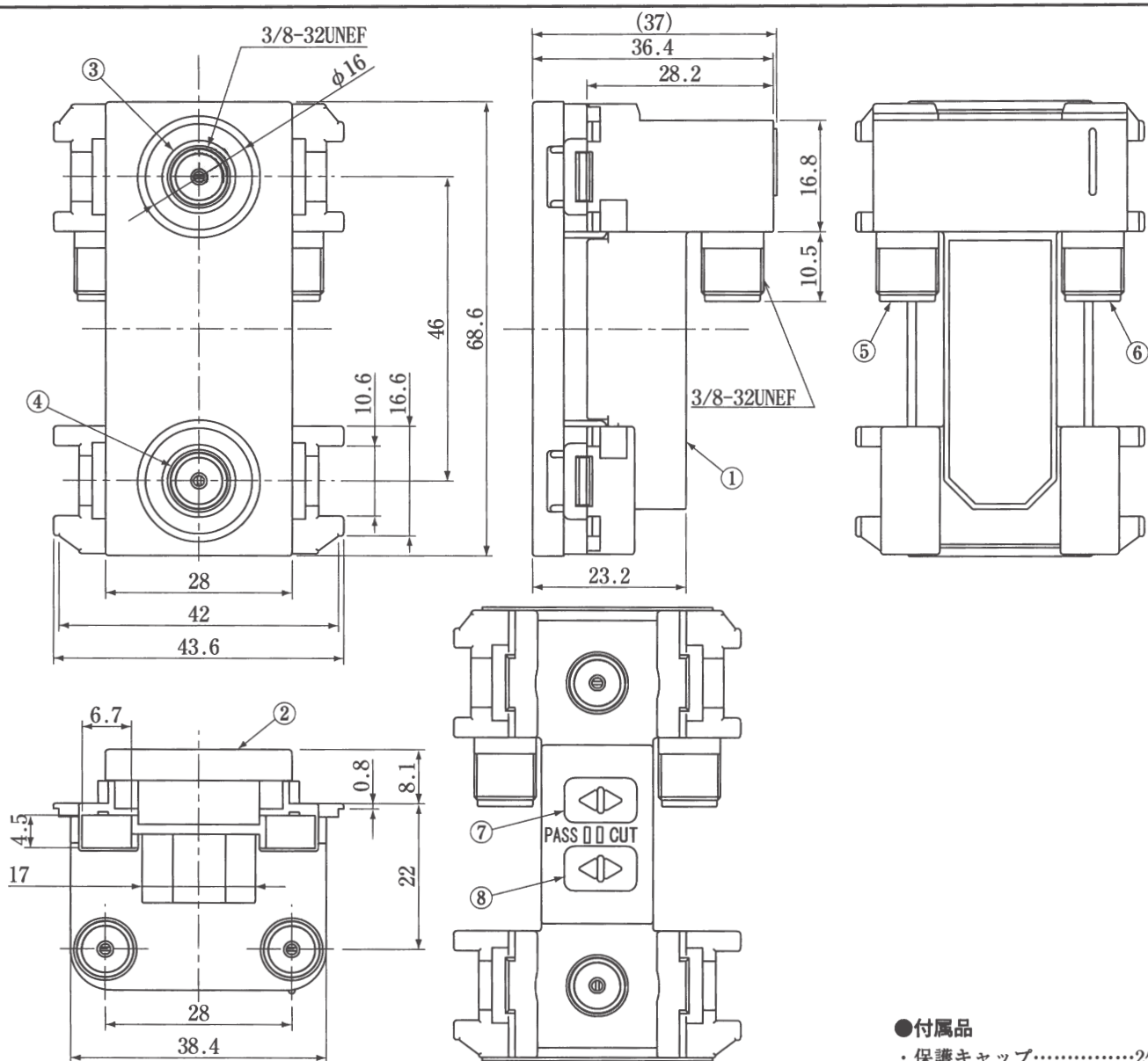
パネル未装着状態図
