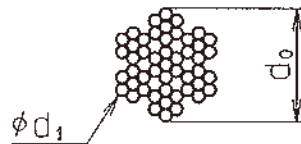
断面 (5: 1)
