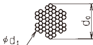
断面 (5: 1)
