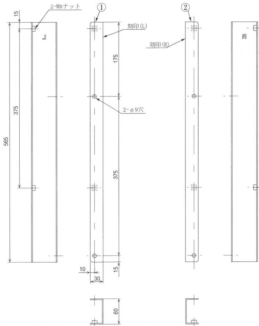
金具R(金具Lの鏡面对象品)
