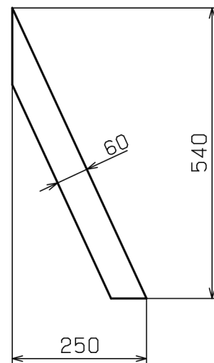
リブ詳細 t 6
