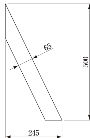
リブ詳細 t6
