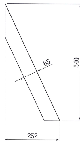
リブ詳細 t6
