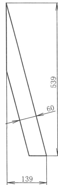
リブ詳細 t6
