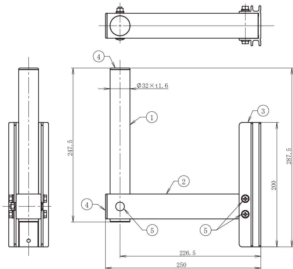
取付金具寸法図
