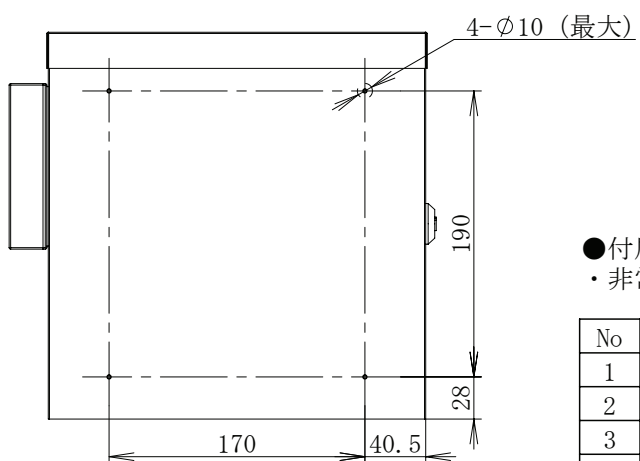
キャビネット穴あけ加工位置
