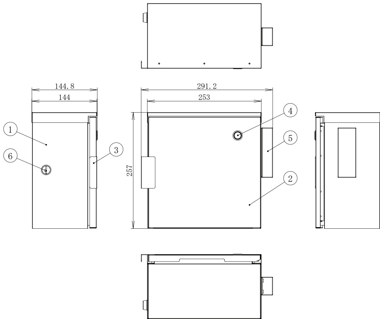
キャビネット穴あけ加工位置
