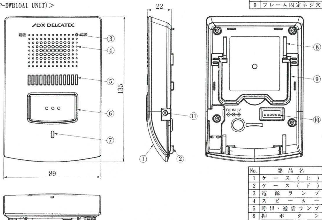
< 親機 (RP-DWB10A1 UNIT) >
