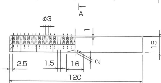
B-B断面図
