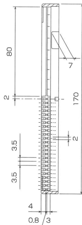
A-A断面図
