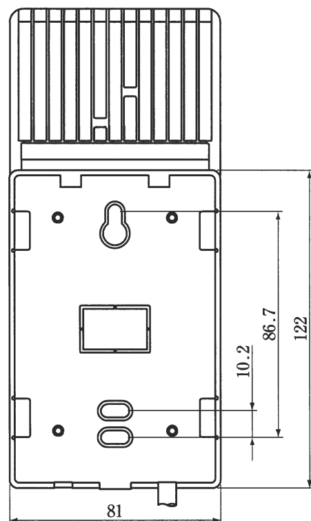
背面
