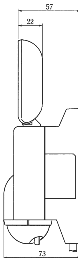
側面
