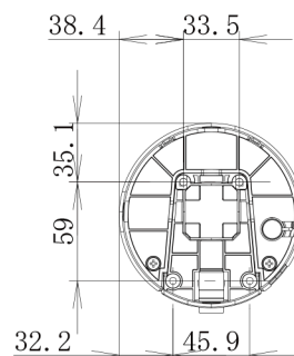
取付ベース詳細 製品内側 (壁面取付用穴の位置)
