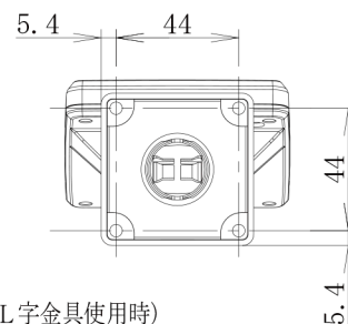
取付ベース詳細 製品内側 (壁面取付用穴の位置) スケール 1:3
