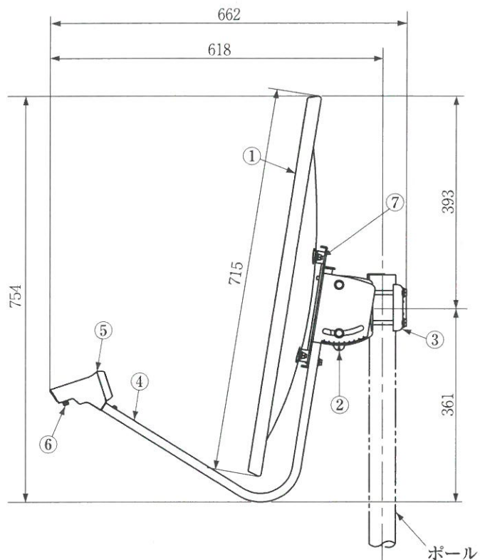
側面
