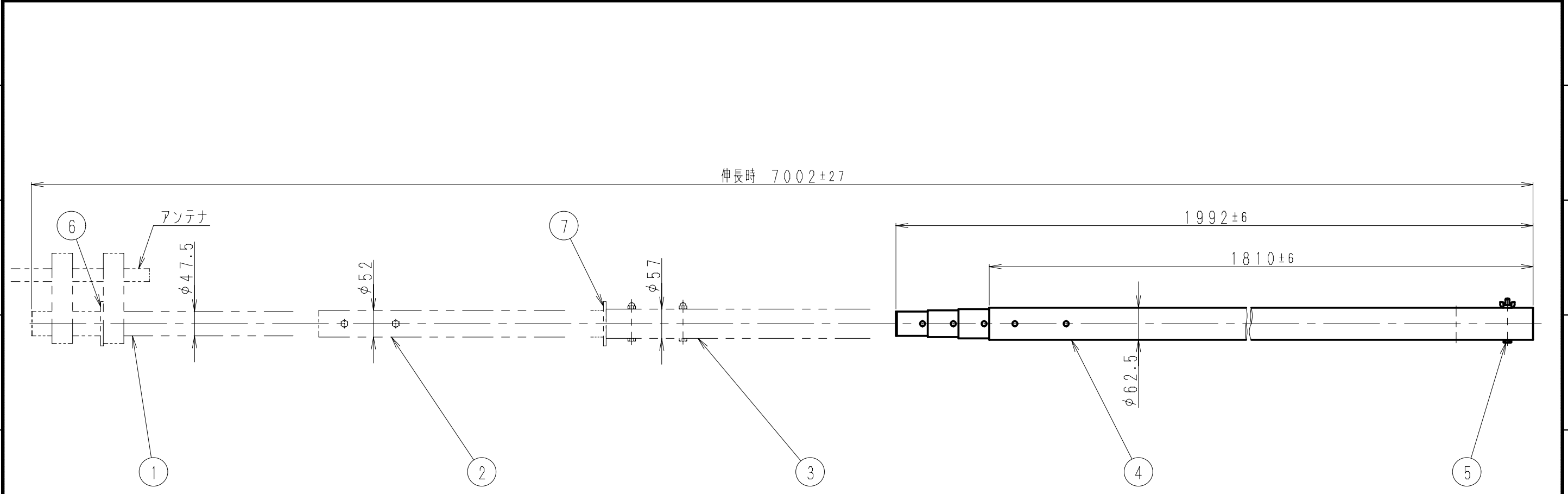
付属品 詳細図 (SCALE 1:5)
