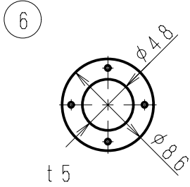
付属品 詳細図 (SCALE 1:5)
