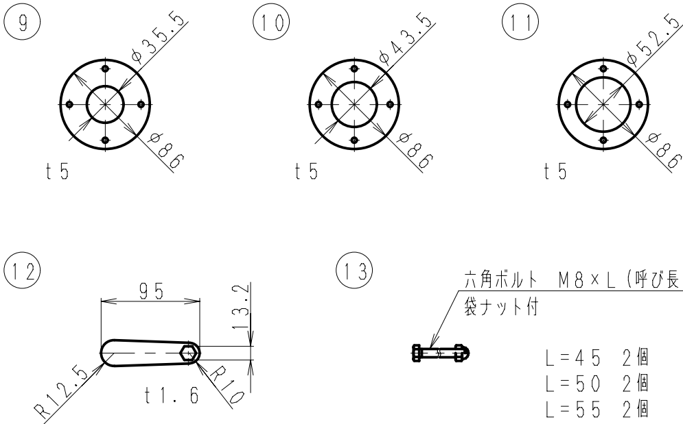
付属品 詳細図 (SCALE 1:5)
