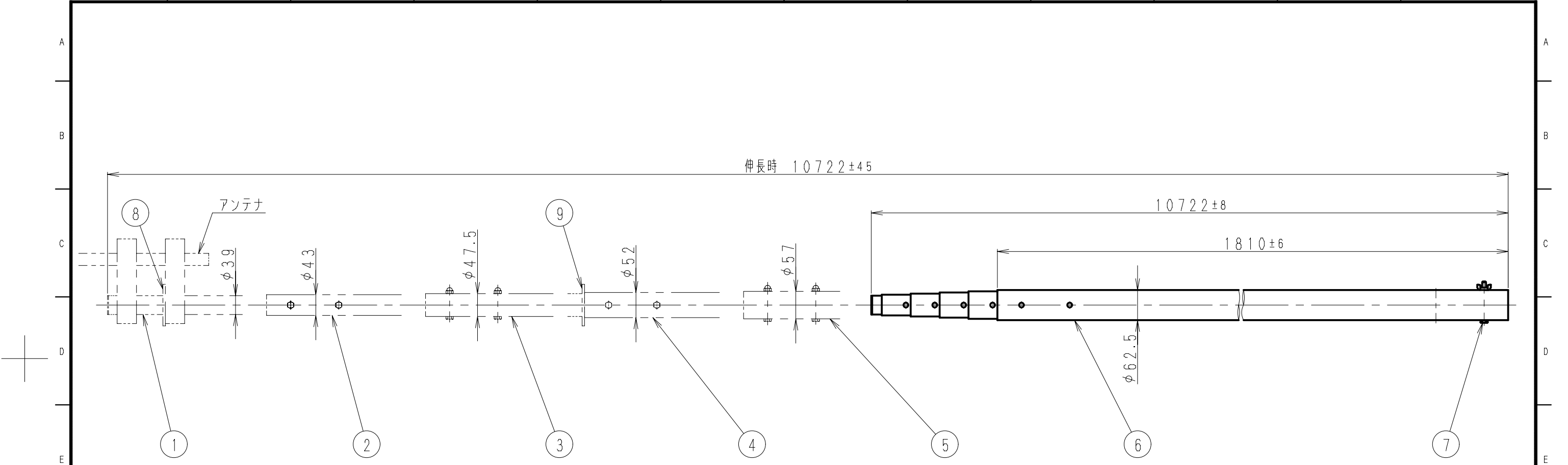
付属品 詳細図 (SCALE 1:5)
