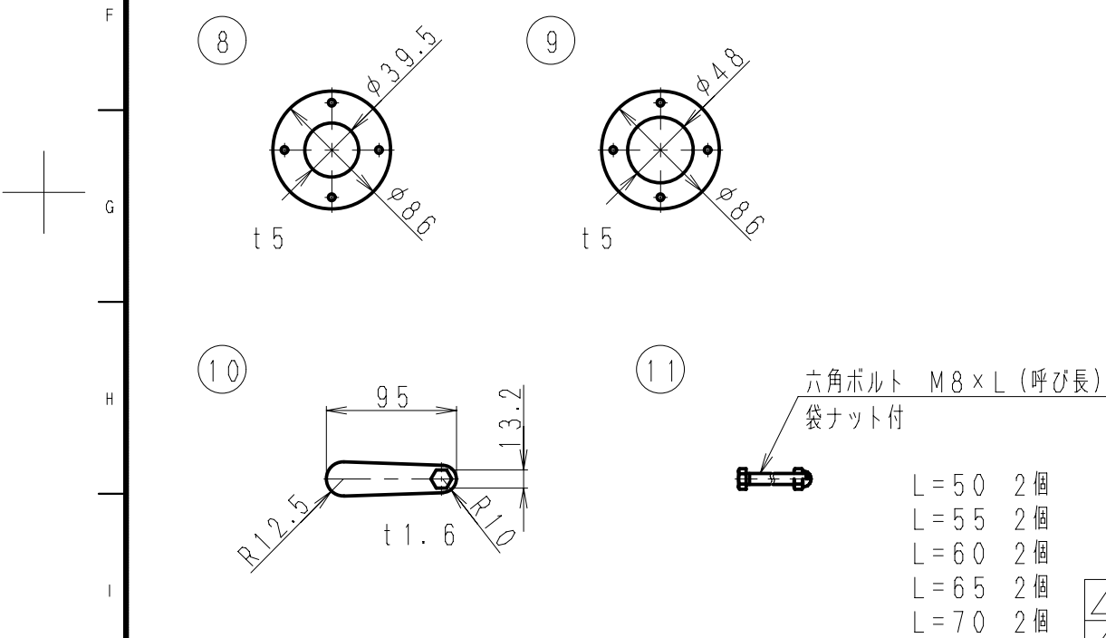
付属品 詳細図 (SCALE 1:5)
