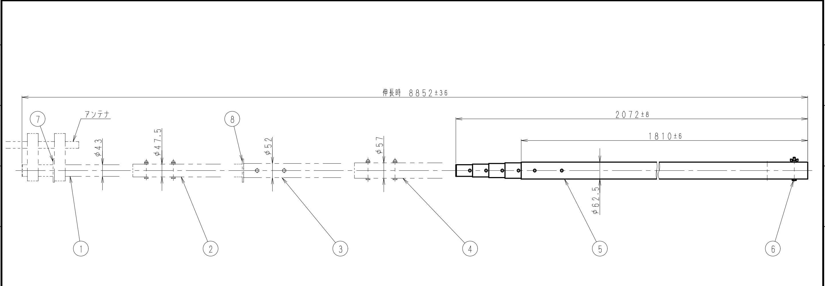
付属品 詳細図 (SCALE 1:5)
