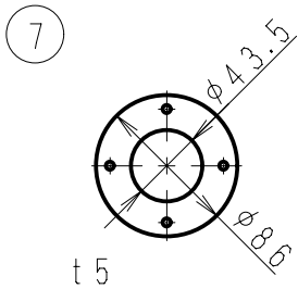
付属品 詳細図 (SCALE 1:5)
