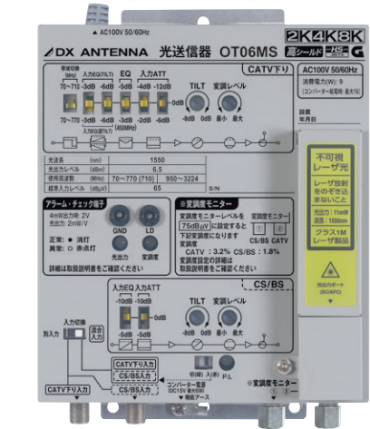
1550nm帯棟内用光送信器 [2K・4K・8K対応]
