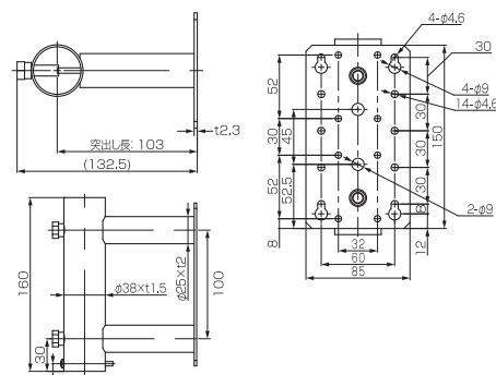
寸法図(mm)
